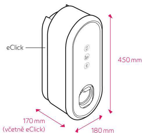
eBox smart se zásuvkou Typu 2
